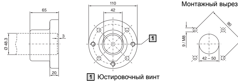
1 Юстировочный винт
