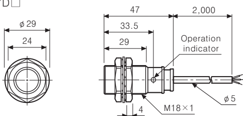
●PRD18-14D□
